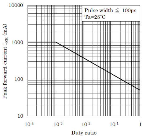
Fig.5 セン頭順電流－デューティ比
